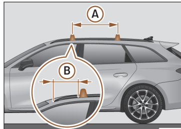
Fig. 192 Puntos de fijación de las barras longitudinales para el portaequipajes del techo (Leon Sportstourer).
