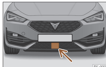
Fig. 121 En el paragolpes delantero: sensor de radar.
