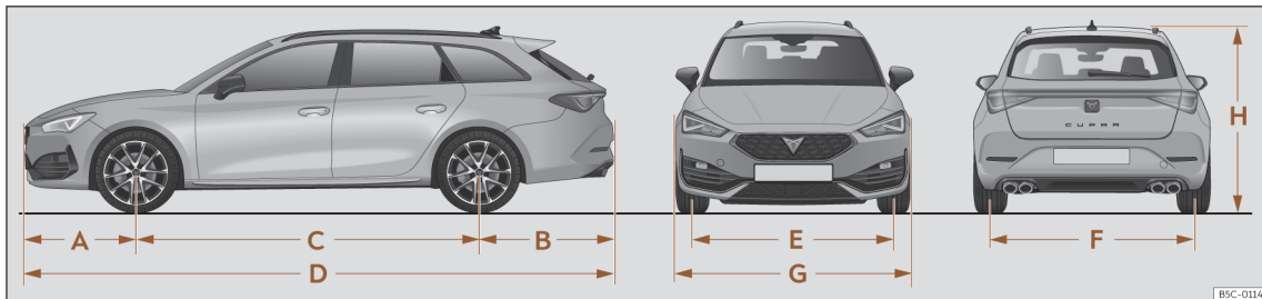
Fig. 240 Dimensiones
